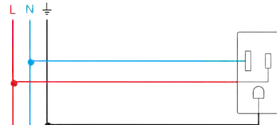
Toma de corriente 2p+tierra
