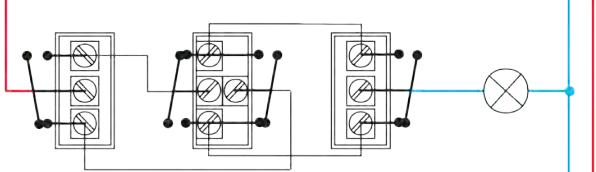
Interruptor 4 vías
