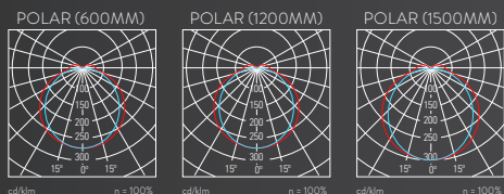
— C0 - C180 — C90 - C270 Curvas fotométricas correspondiente a 4000K.
