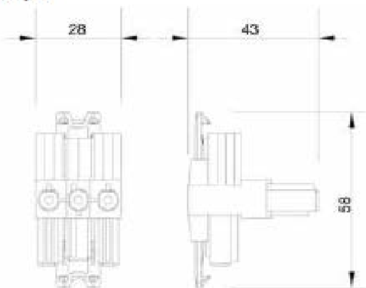
Рисунок 1. СИСТЕМА БЫСТРОГО СИЛОВОГО ПОДКЛЮЧЕНИЯ (СБСП)
